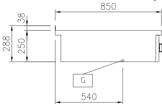
Zij aanzicht
